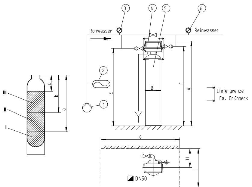
Abb. 2: Aufstellungszeichnung mit Fundamentplan
